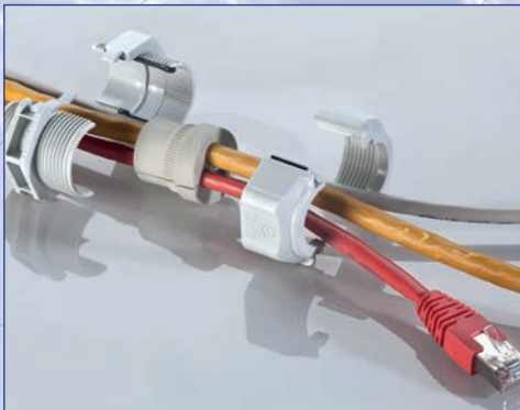
Teilbare Kabelverschraubung UNI Split Gland Splittable cable gland UNI Split Gland Presse-étoupe divisible UNI Split Gland
