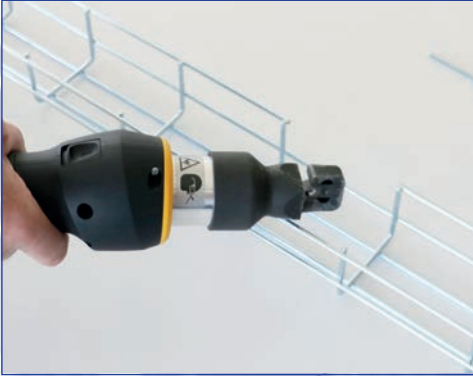
Mobile Gitterkanalschere Portable wire tray shears Tenaille mobile pour canivaux à grille
