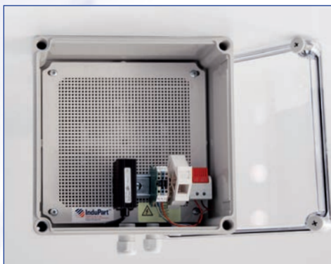
WLAN Schutzgehäuse mit oder ohne Heizung Junction box WLAN with or without heating Boîte de protection WLAN avec ou sans chauffage
