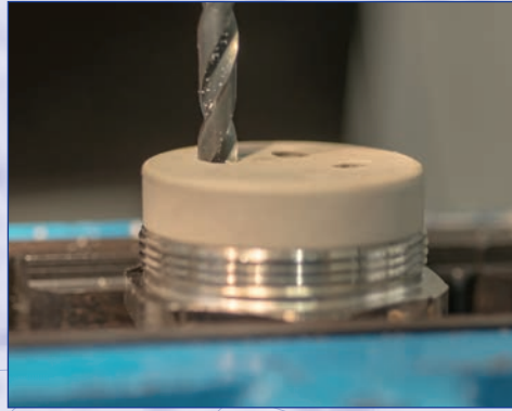
Bohren von Dichteinsätzen Drilling of inserts for cable glands Perforation d'inserts pour presse-étoupes
